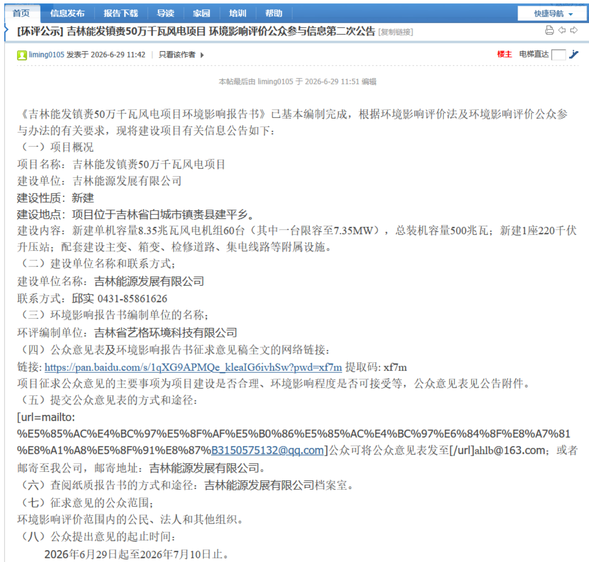
图 3.2-1 网页截图
